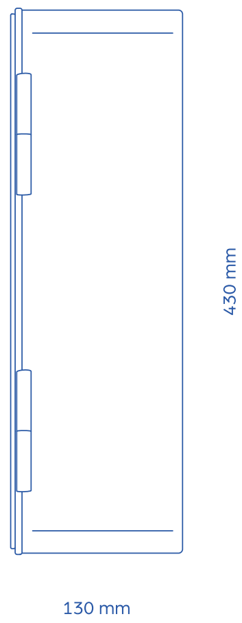
Schématický bokorys
